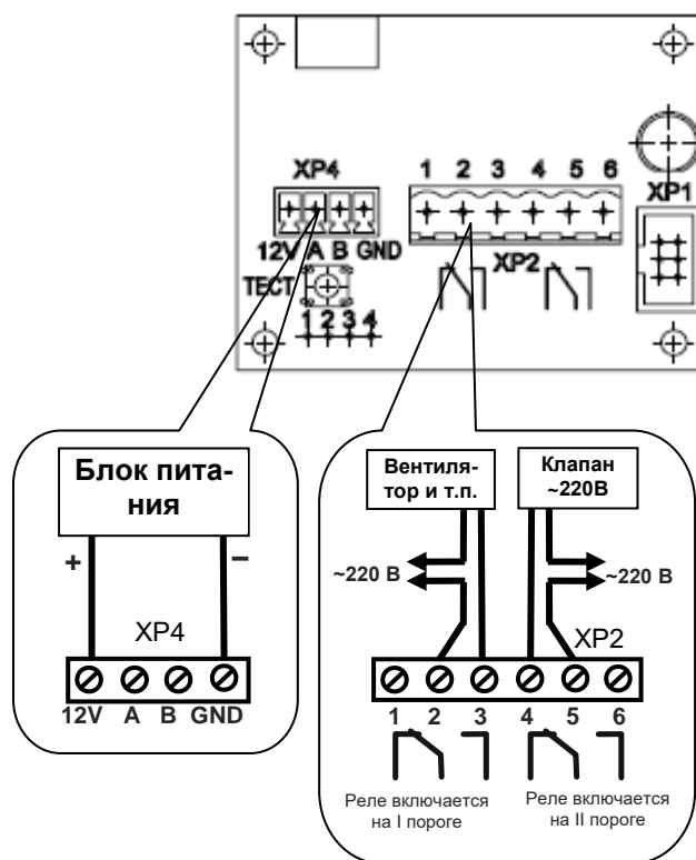
Рисунок 6 – Схема соединения оборудования с двухблочным Сигнализатором
