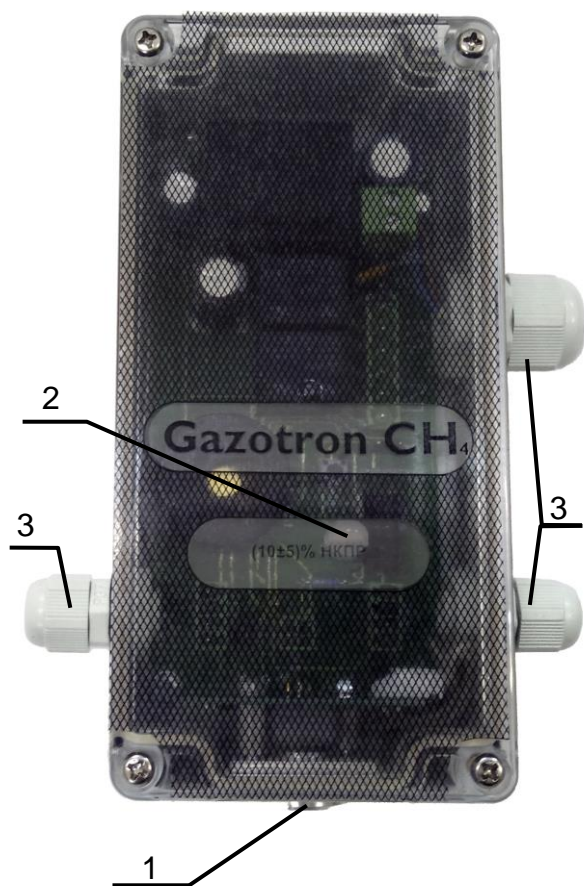
1 – датчик; 2 – светодиод; 3 – гермовводы
